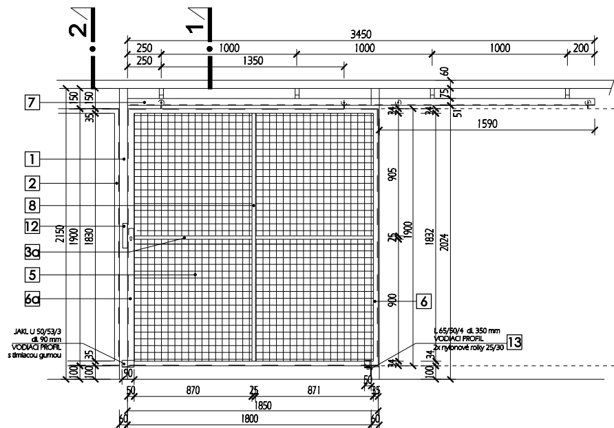
POHĽAD NA ZASÚVACIU BRÁNU
