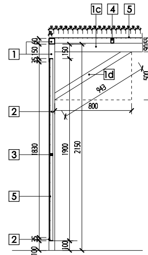
PRIEČNÝ REZ
